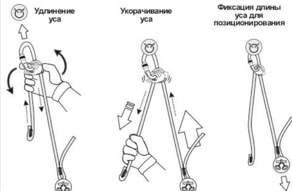
Рис. 9. Регулировка длины уса самостраховки в процессе использования
