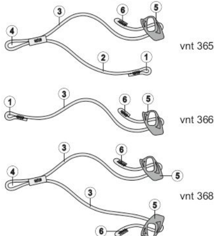
Рис. 1. Внешний вид, состав усов самостраховки
